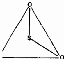
4.12 Sulphur dioxide e.
